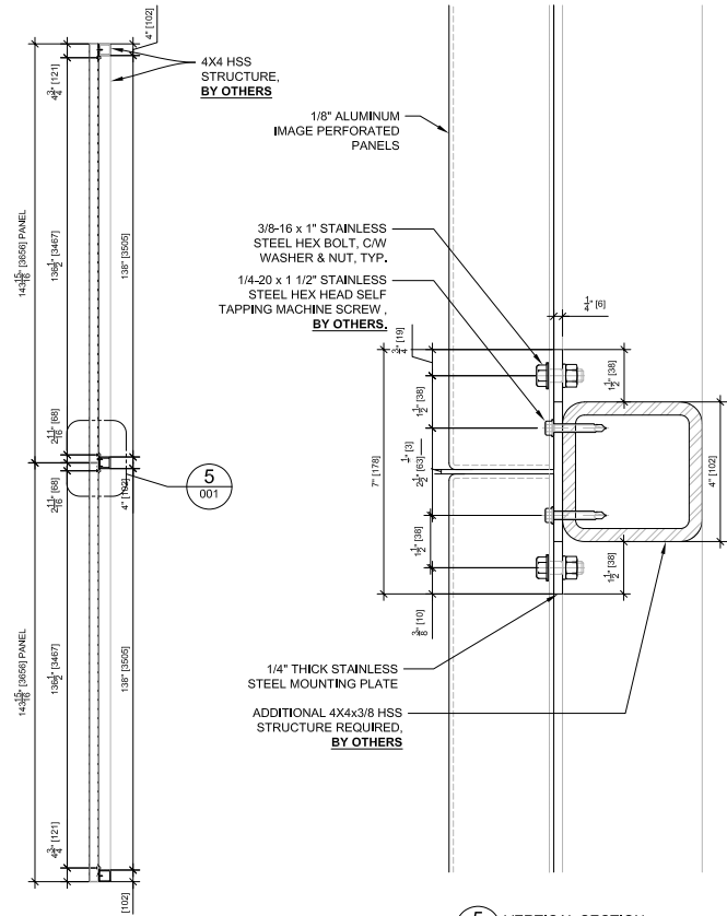
4 VERTICAL SECTION 001 SCALE: 1/2" = 1'-0"
