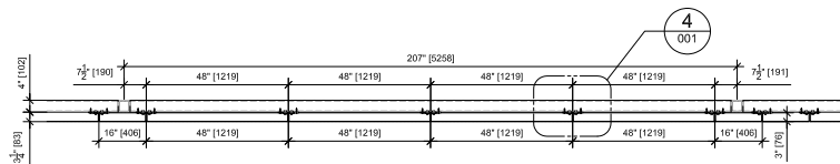
2 HORIZONTAL SECTION 001 SCALE: 1/2" = 1'-0"
